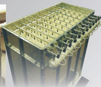
Filtro a maniche autopulente
